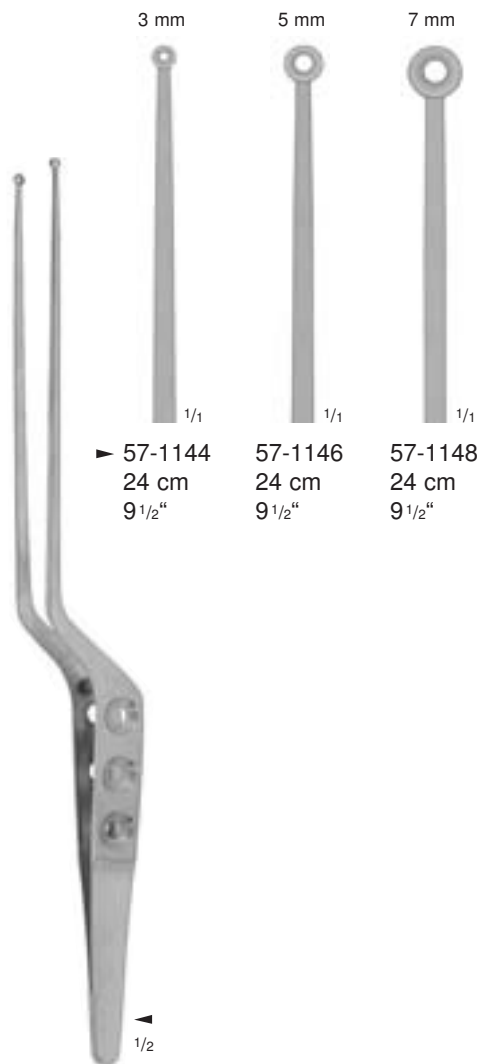
YASARGIL-SAMII 57-1144 - 57-1148 Maul löffelförmig jaws spoon-shaped boca forma cuchara Mors en forme de cuillère Morsi a forma di cucchiaio
